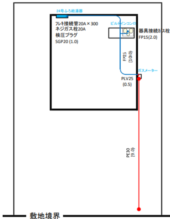
内管工事見積平面図
