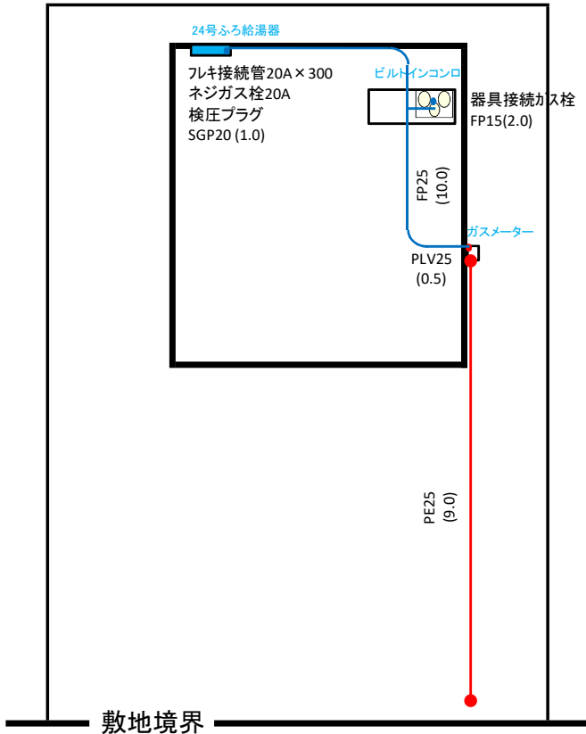
内管工事見積平面図
